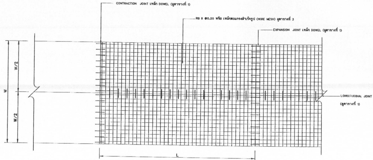
แปลนแสดงการเสริมเหล็กถนน ค.ค.ล.
