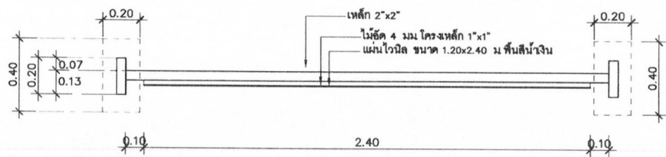
แปลน 1:20
