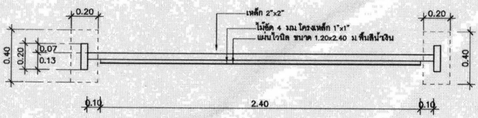
แปลน 1:20
