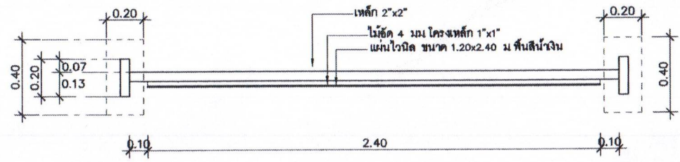
แปลน 1:20
