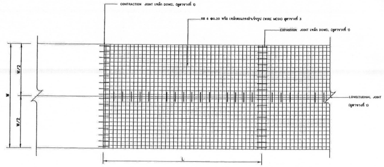
แบบแผนผังการเสริมเหล็กถนน ค.ค.ค.
