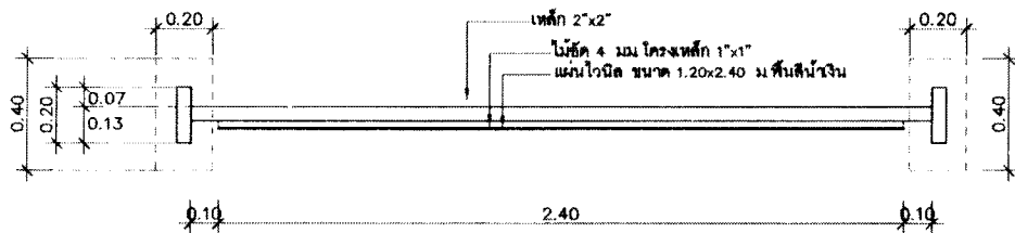
แปลน 1:20
