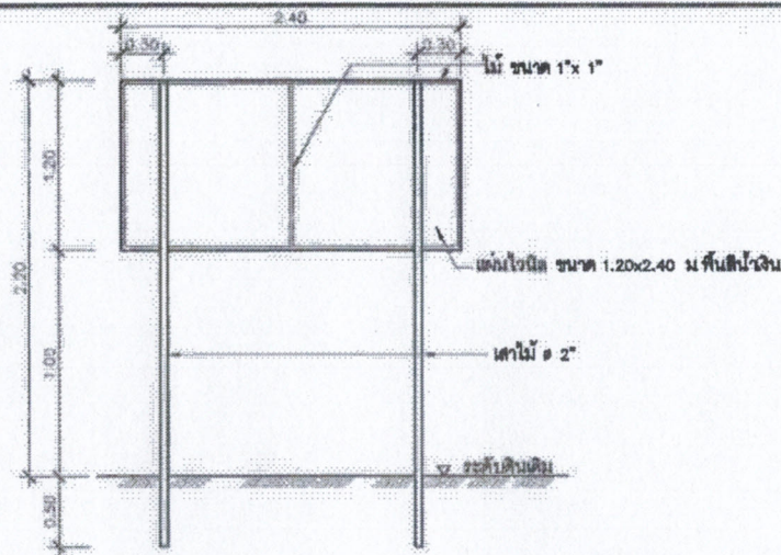
แบบโครงสามพื้นโครง
