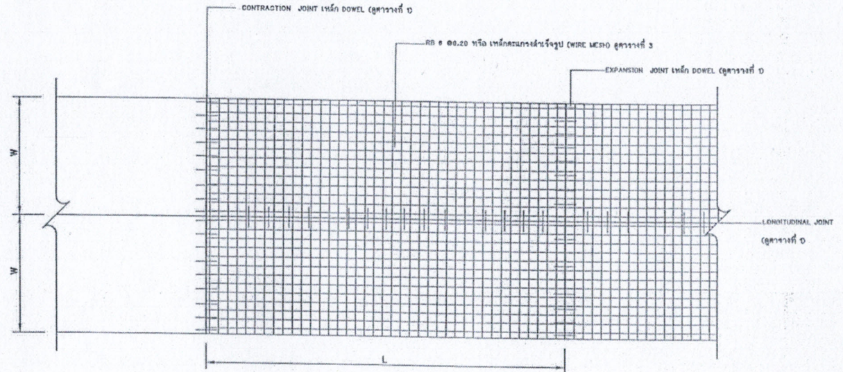
แปลนแสดงการเสริมเหล็กถนน ค.ค.ล.
