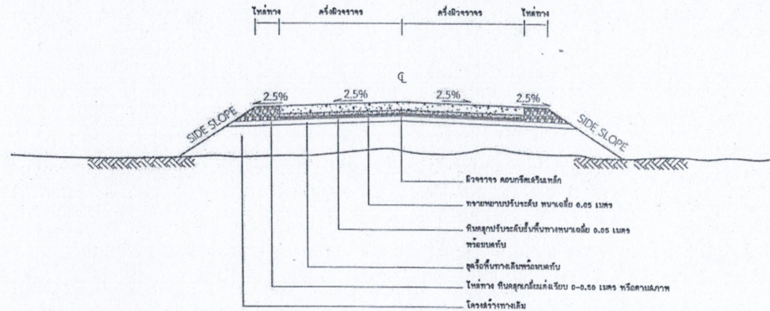
รูปตัดแฉะ โครงสร้างถนนคอนกรีตเสริมเหล็กและคูน้ำบดผิว
