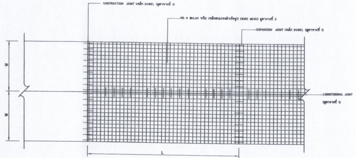
แบบแปลนแสดงการเสริมเหล็กถนน ค.ล.ล.
