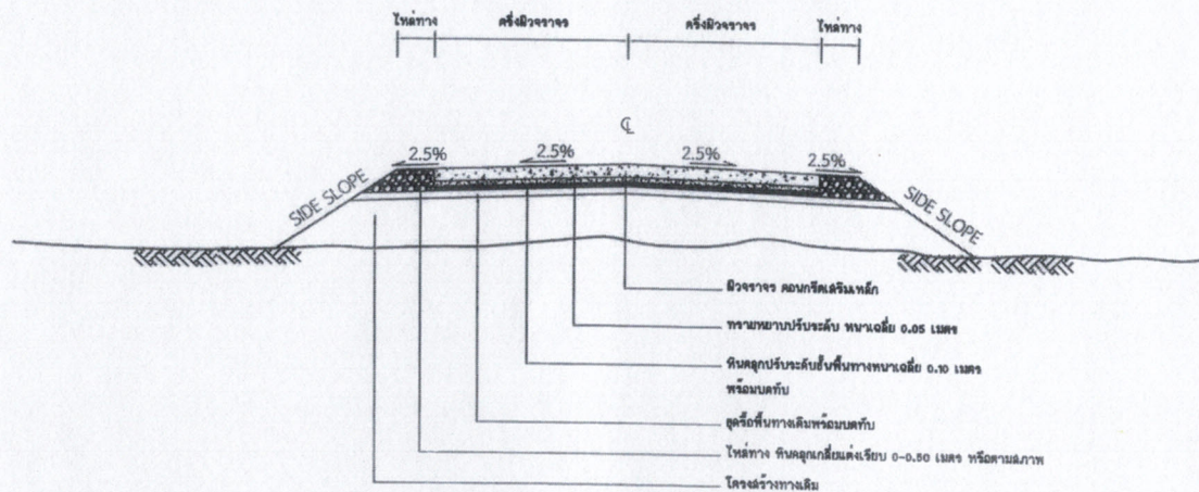
รูปตัดแลดงโครงสร้างถนนคอนกรีตเสริมเหล็กและคุณสมบัติวัสดุ
