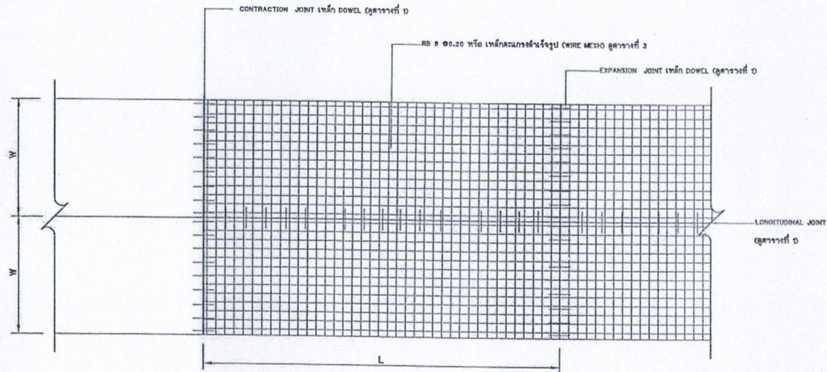
แปลนแสดงการเสริมเหล็กถนน ค.ฉ.ล.
