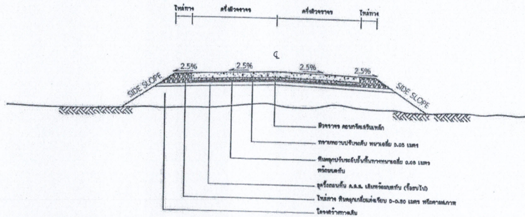
รูปตัดแสดงโครงสร้างถนนคอนกรีตเสริมเหล็กและคลุมมบิวดิว
