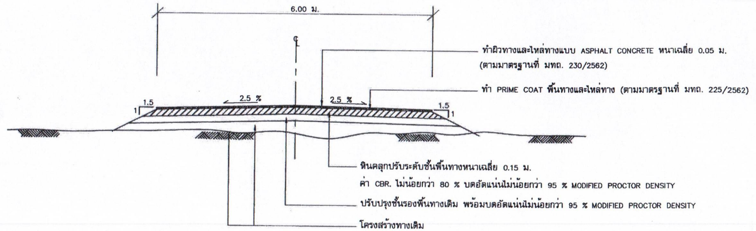
รูปตัดโครงสร้างทางผิวจราจรแบบ ASPHALT CONCRETE กม.1+200 ถึง กม.2+100
