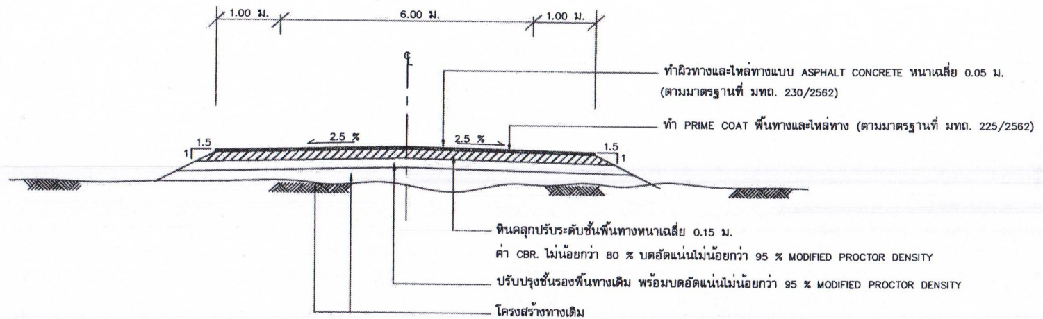
รูปตัดโครงสร้างทางผิวจราจรแบบ ASPHALT CONCRETE กม.3+100 ถึง กม.4+800
