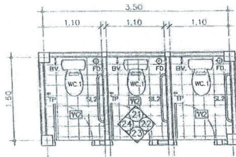
แปลนห้องน้ำชาย มาตราส่วน 1:50
