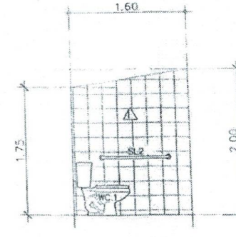
รูปด้าน 22 มาตราส่วน 1:50
