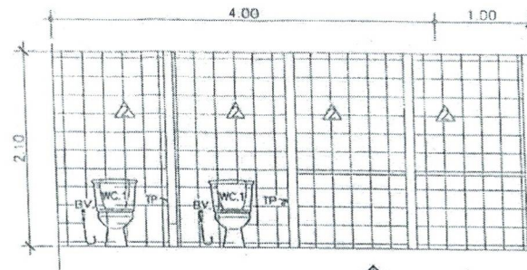
รูปด้าน 15 มาตราส่วน 1:50
