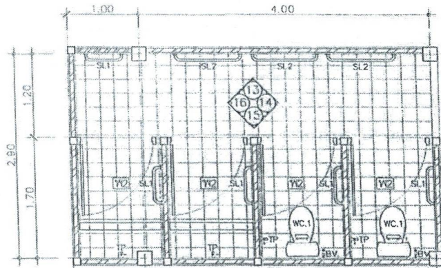
แปลนห้องน้ำอาคารเรือนนอนหญิง 2 มาตราส่วน 1:50
