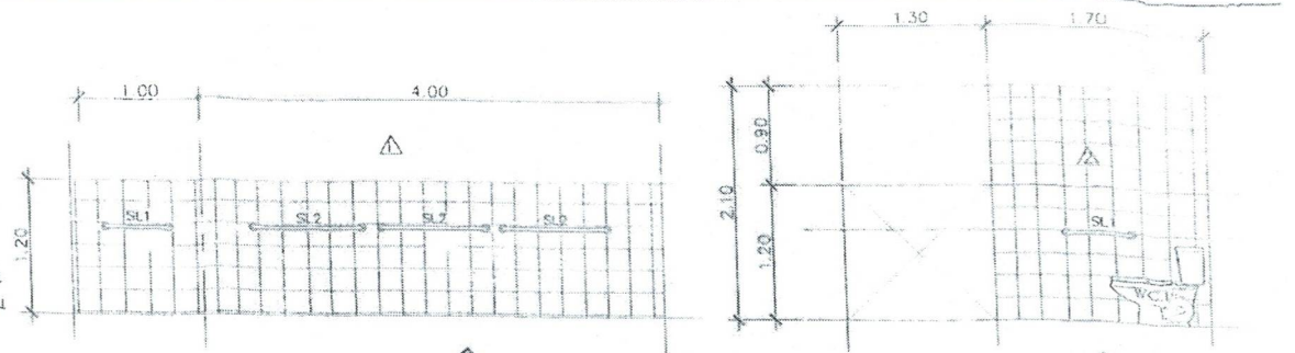
รูปด้าน 13 มาตราส่วน 1:50
