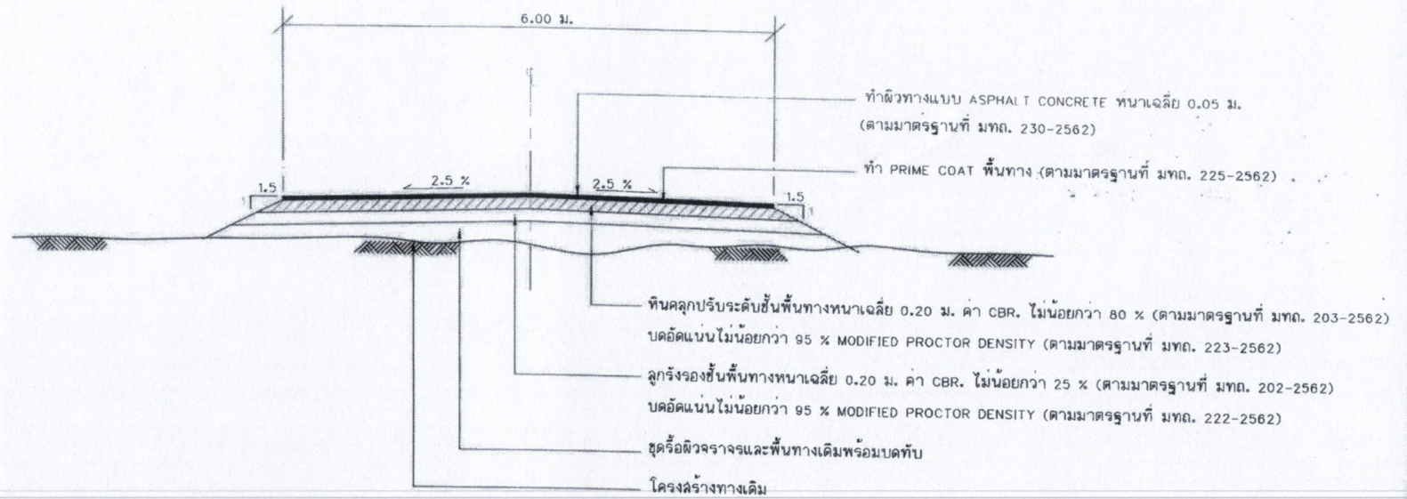
รูปตัดโครงสร้างทางผิวจราจรแบบ ASPHALT CONCRETE (ช่วง กม.ที่ 0+000 ถึง กม.ที่ 0+430)
