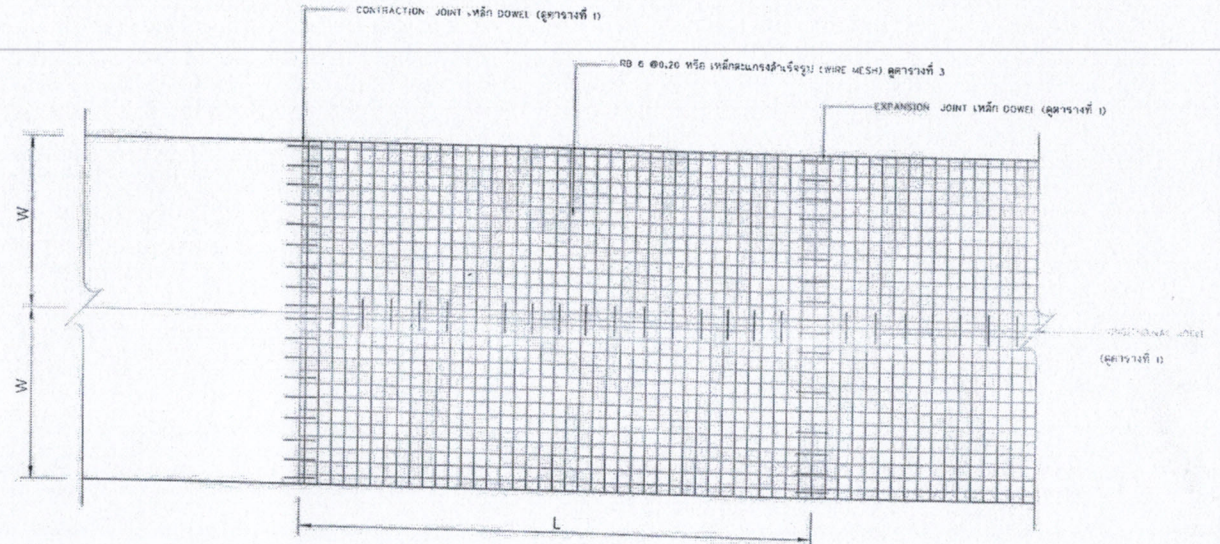
แบบแปลนแสดงการเสริมเหล็กถนน ค.ฉ.ฉ.
