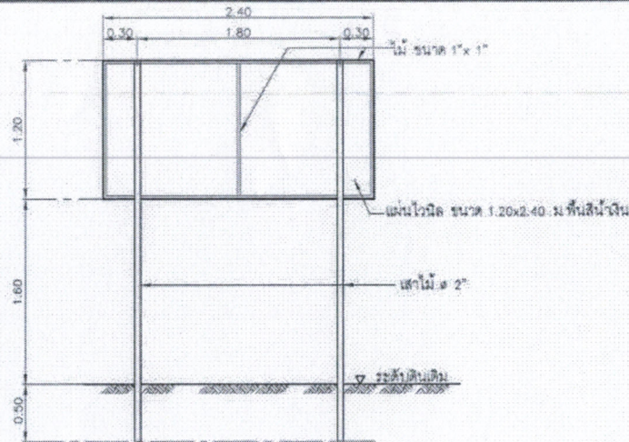
แบบแสดงการปักป้ายชั่วคราว
