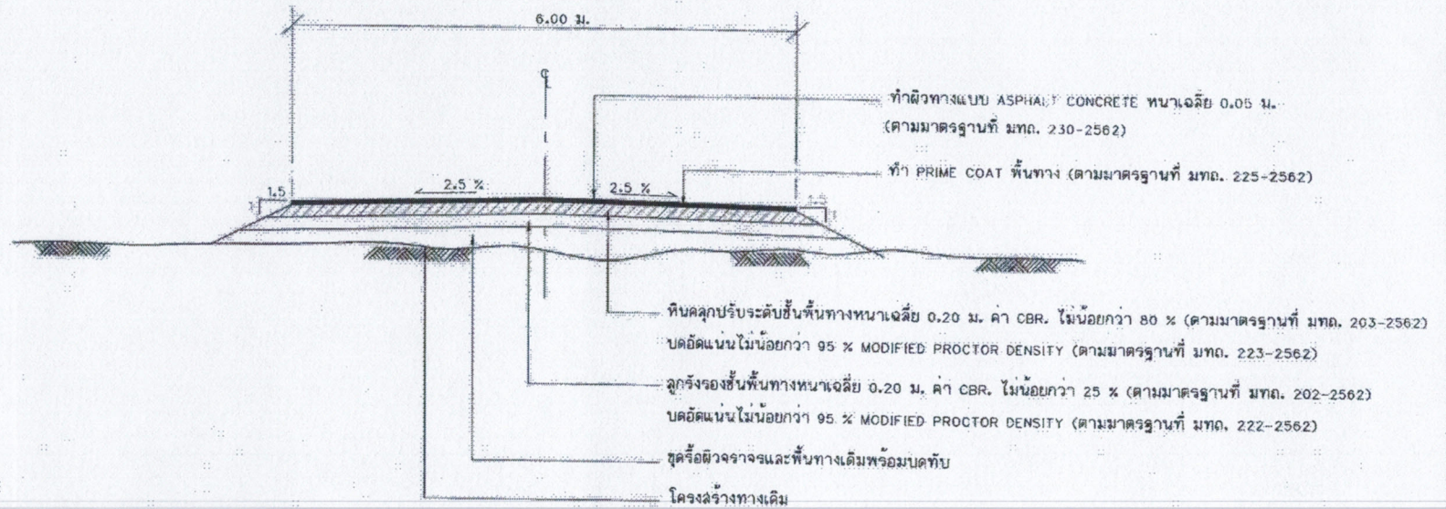
รูปตัดโครงสร้างทางผิวจราจรแบบ ASPHALT CONCRETE (ช่วง กม.ที่ 0+000 ถึง กม.ที่ 1+070)
