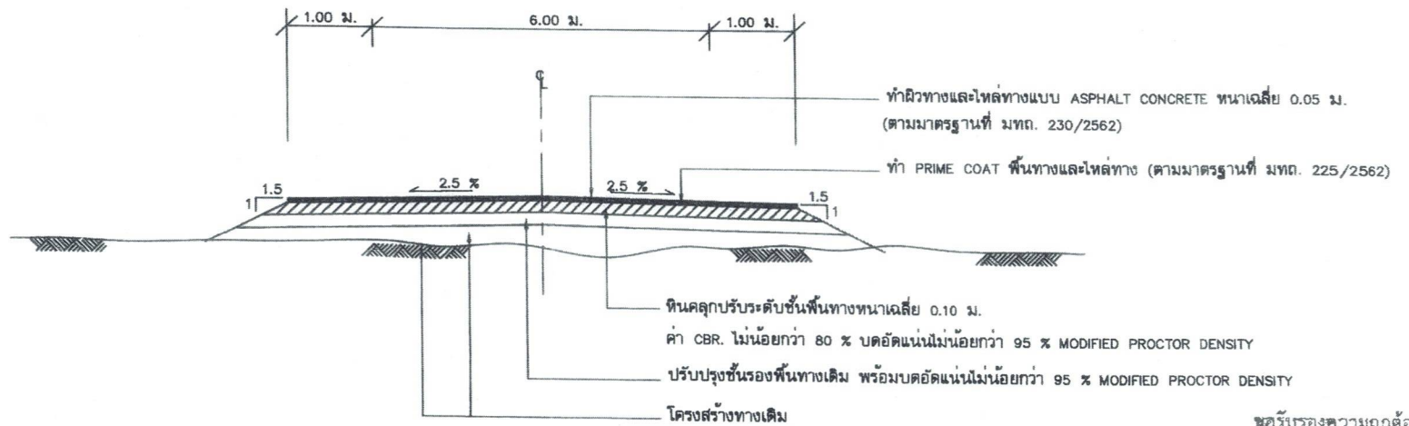
รูปตัดโครงสร้างทางผิวจราจรแบบ ASPHALT CONCRETE กม.ที่ 3+900 ถึง กม.ที่ 4+500
