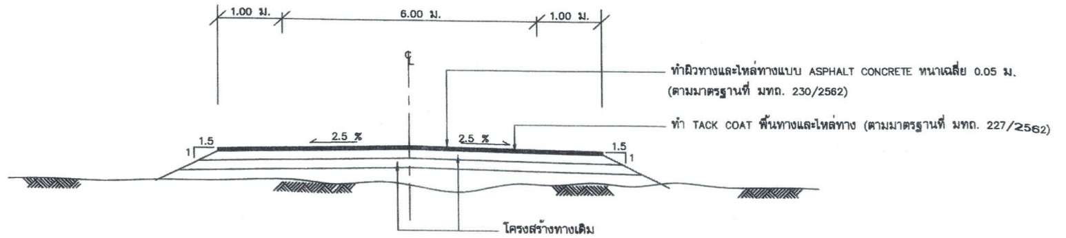
รูปตัดโครงสร้างทางผิวจราจรแบบ ASPHALT CONCRETE กม.ที่ 0+400 ถึง กม.ที่ 1+200
