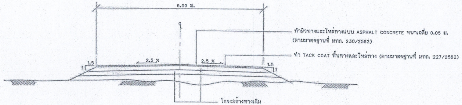
รูปตัดโครงสร้างทางผิวจราจรแบบ ASPHALT CONCRETE มาตรฐาน 1 : 75
