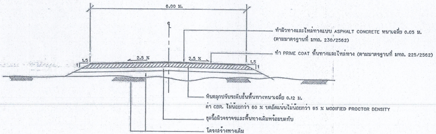
รูปตัดโครงสร้างทางผิวจราจรแบบ ASPHALT CONCRETE มาตรฐาน 1 : 75
