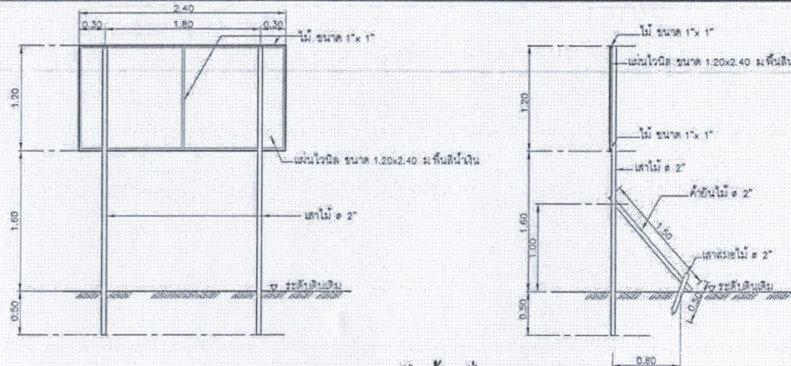
แบบแสดงการปักป้ายชั่วคราว
