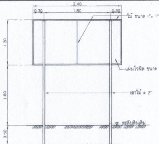
แบบแสดงการปักป้ายชั่วคราว
