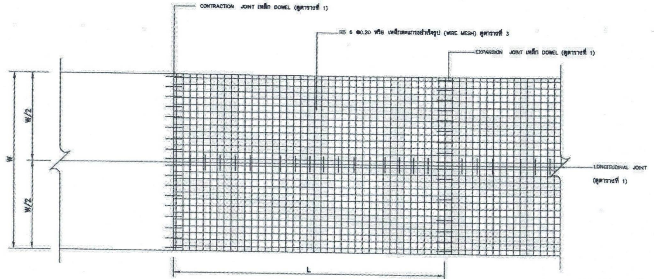
แบบแปลนแสดงการเสริมเหล็กคอนกรีต ค.ส.ล.
