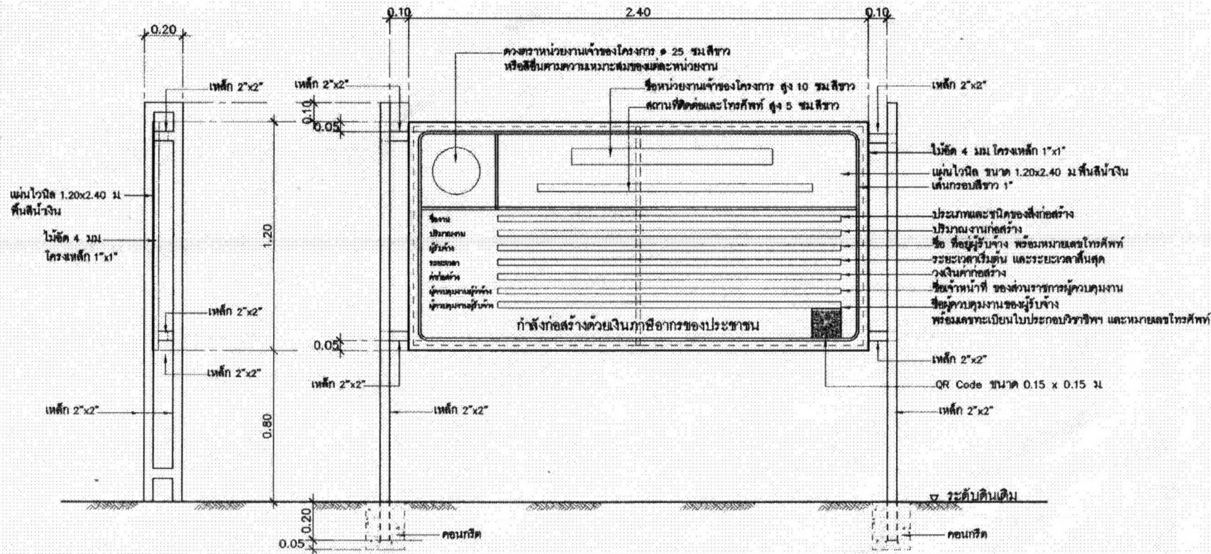
รูปด้านหน้า 1:20
