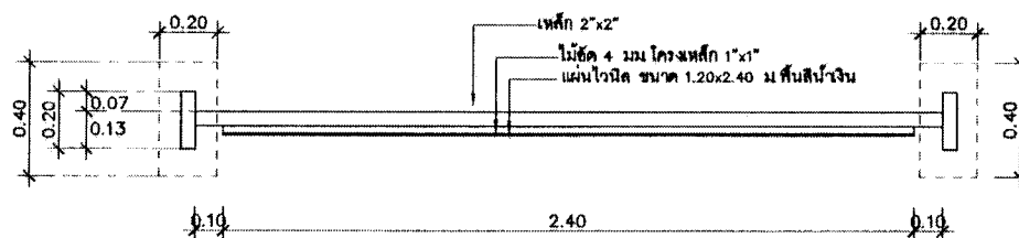
แปลน 1:20
