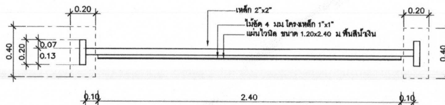
แปลน 1:20
