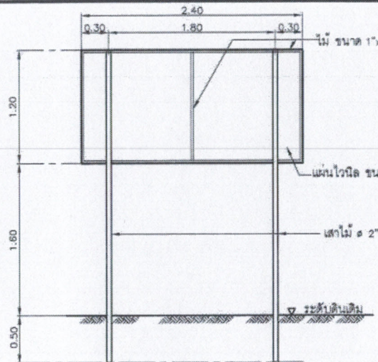
แบบแสดงการปักป้ายชั่วคราว
