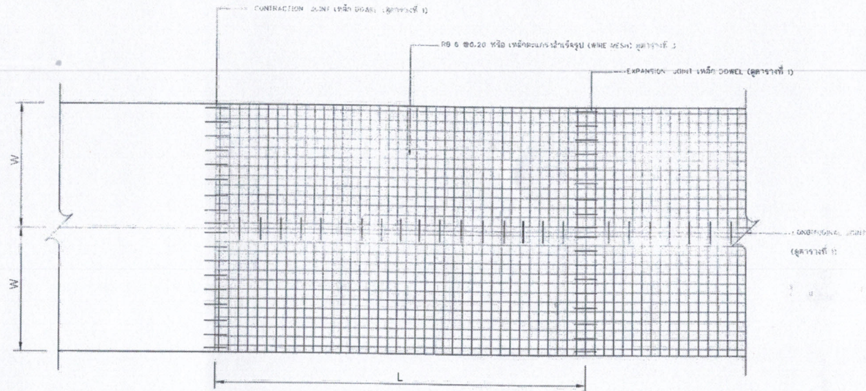
แบบแผนแสดงการเสริมเหล็กถนน ค.ล.ล.
